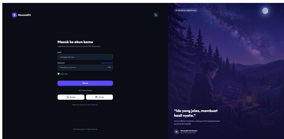
Gambar 3. Halaman Login.
